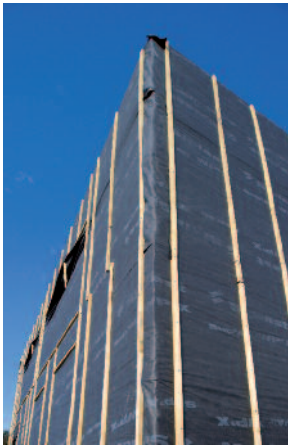
Pose sur chantier de la maison à ossature bois BBC Maison LY, http://www.maison-respekt.fr/projets/maison+ly , Photos Dominique Eskenazi pour Siplast.
