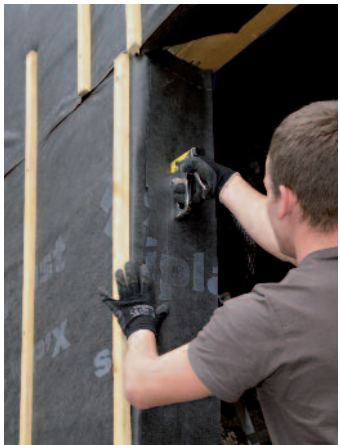
Pose sur chantier de la maison à ossature bois BBC Maison LY, http://www.maison-respekt.fr/projets/maison+ly , Photos Dominique Eskenazi pour Siplast.
